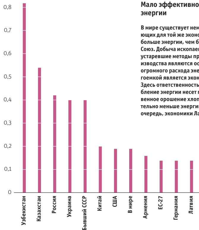
Кол-во израсходованных единиц топлива в тоннах в расчете на валовую добавленную стоимость в размере 1.000 долларов США (2000 г.) по паритету покупательной способности
